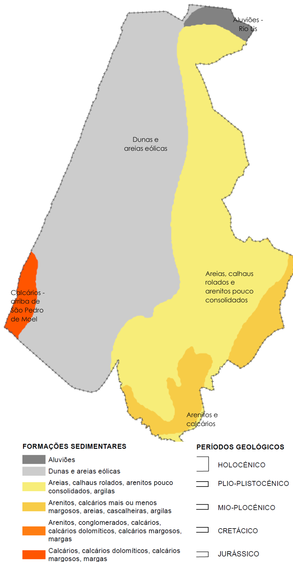
Figura 1. Litologia no concelho da Marinha Grande
