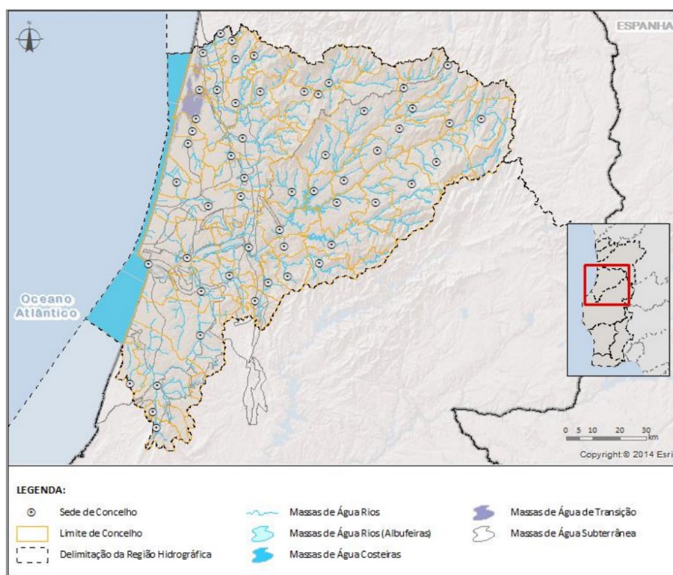
Figura 74. Delimitação geográfica da Região Hidrográfica do Vouga, Mondego e Lis
